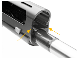
Lubrique levemente los rieles del cerrojo dentro del cajón de mecanismos.
